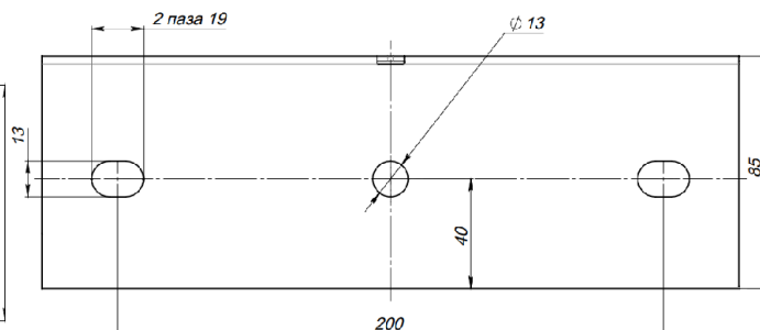
Монтажные отверстия
